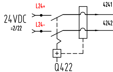
操作台24V电源 Электропитание 24V в панели управления
