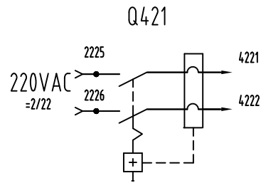
操作台220V电源 Электропитание 220V в панели управления
